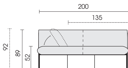
Frontansicht Typ B200FL
